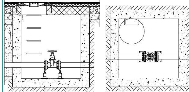
POZZETTO DI ALLOGGIAMENTO SARACINESCA
