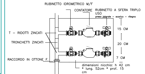
ALLACCIO D'UTENZA -TIPO-
