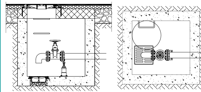
POZZETTO DI SCARICO
