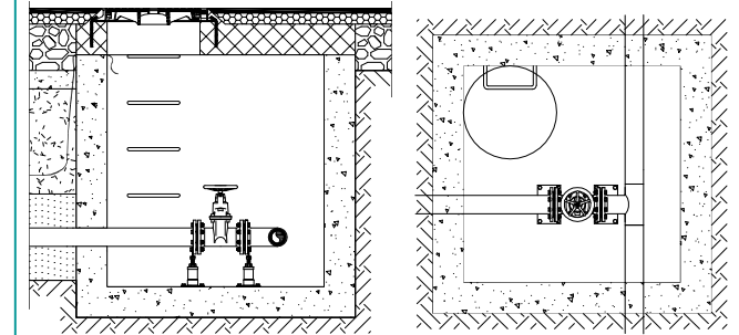
POZZETTO DI ALLOGGIAMENTO SARACINESCA
