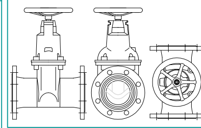
SARACINESCHE CUNEO GOMMATO
