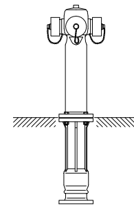
IDRANTE SOPRASUOLO
