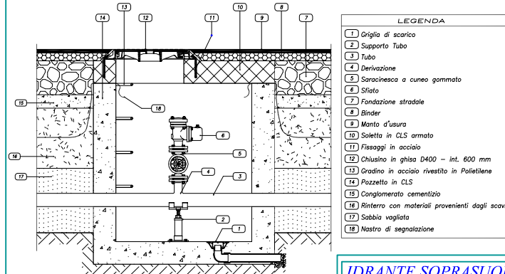
IDRANTE SOPRASUOLO
