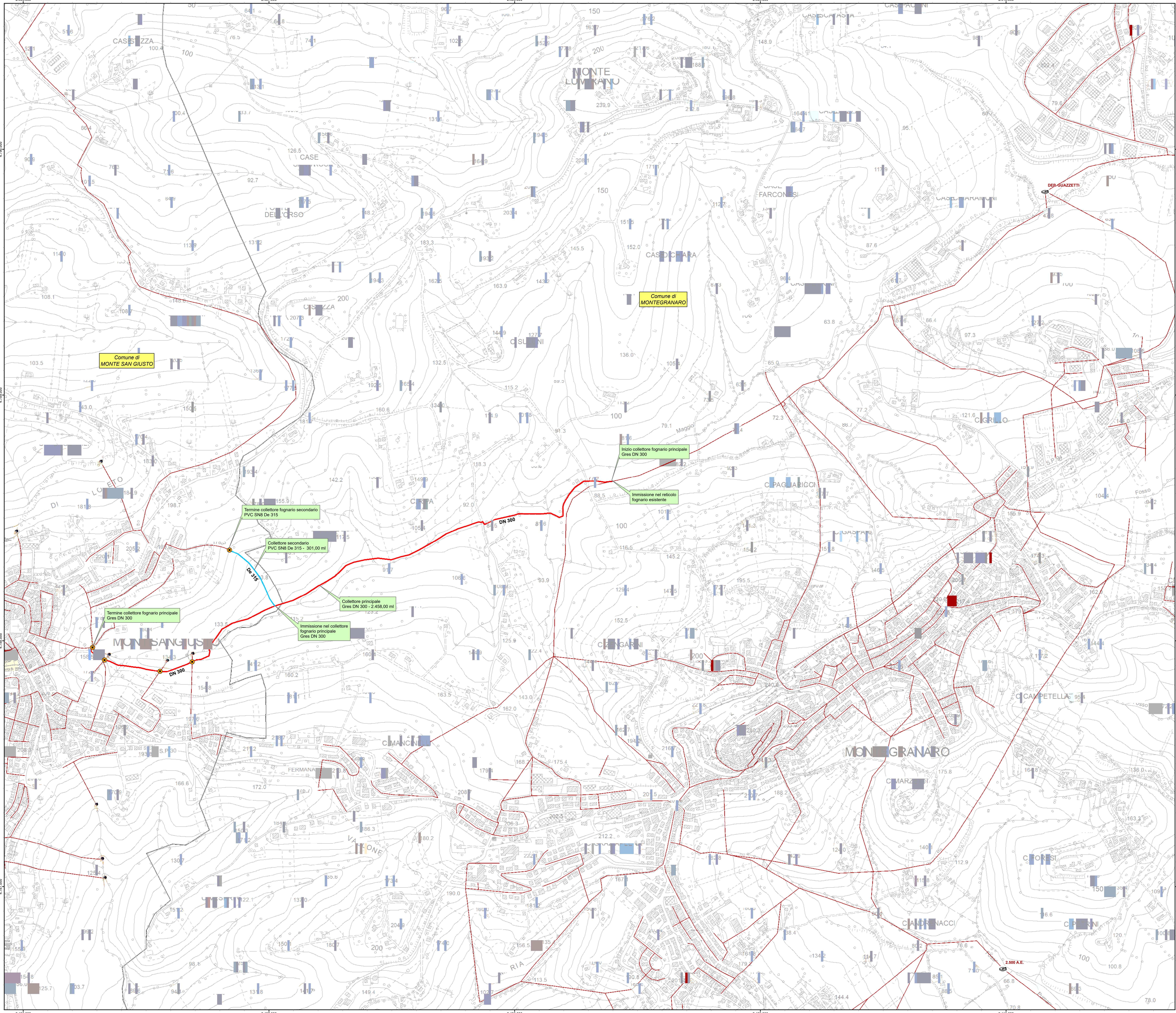
INQUADRAMENTO TAVOLA COROGRAFICA Corografia Collettori fognari principale e secondario
